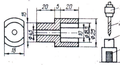
Чертеж кондуктора и сборки деталей для высверливания отверстий в пыжах: 1 — дрель, 2 — сверло диаметром 4,5 мм, 3 — кондуктор, 4 — пыжи
