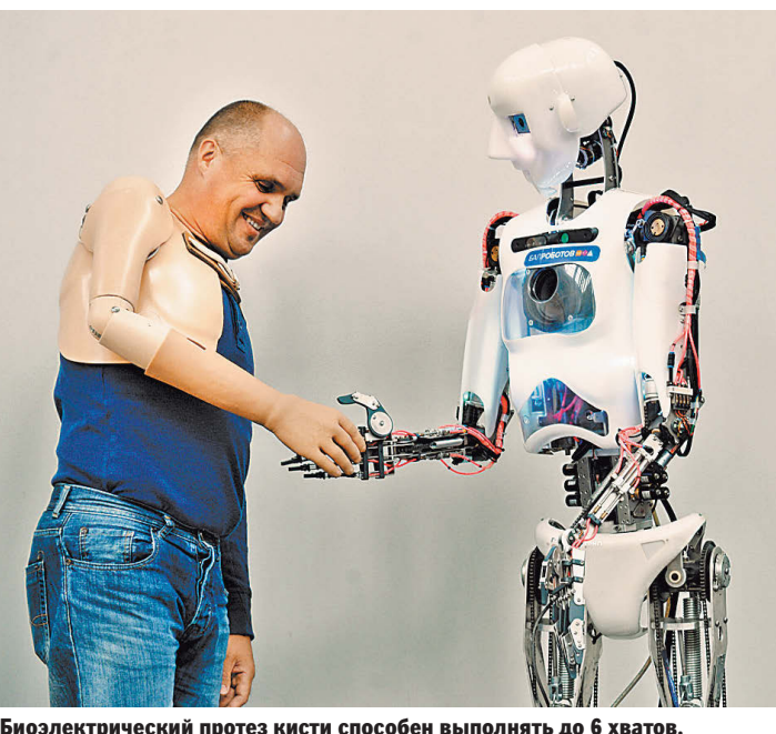
Биоэлектрический протез кисти способен выполнять до 6 хватов.
