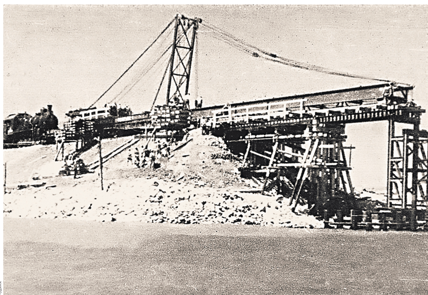
1944 год. Строится первый пролет моста.
