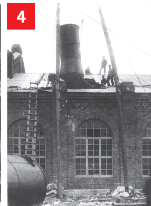
1) ВГЭС № 1 в 1932 году. 2) Кладка дымохода котла на ВГЭС. 3) Кладка котла Фитцнер и Гемпер, 1927 год. 4) Установка трубы на ВГЭС.
