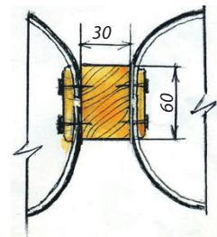
Конструктивный узел мягкой перегородки
