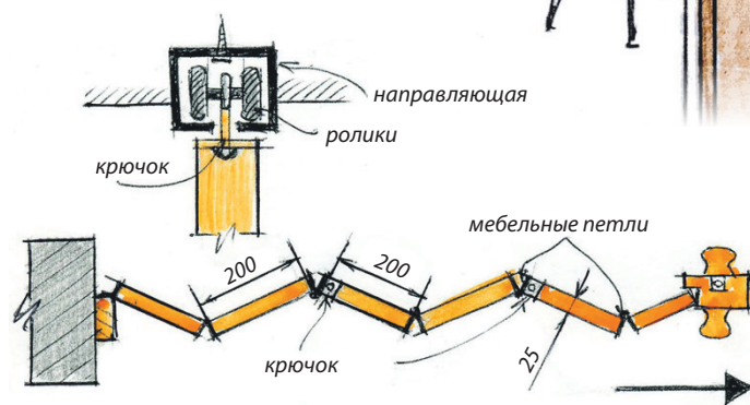
Рис. 4. Раздвижная перегородка
