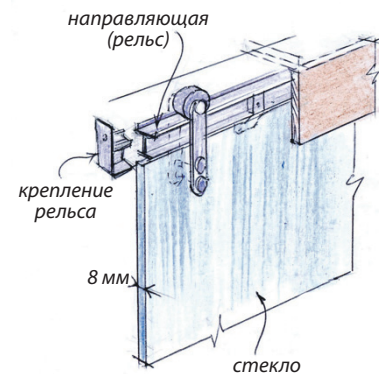
Рис. 6. Стеклопанель
